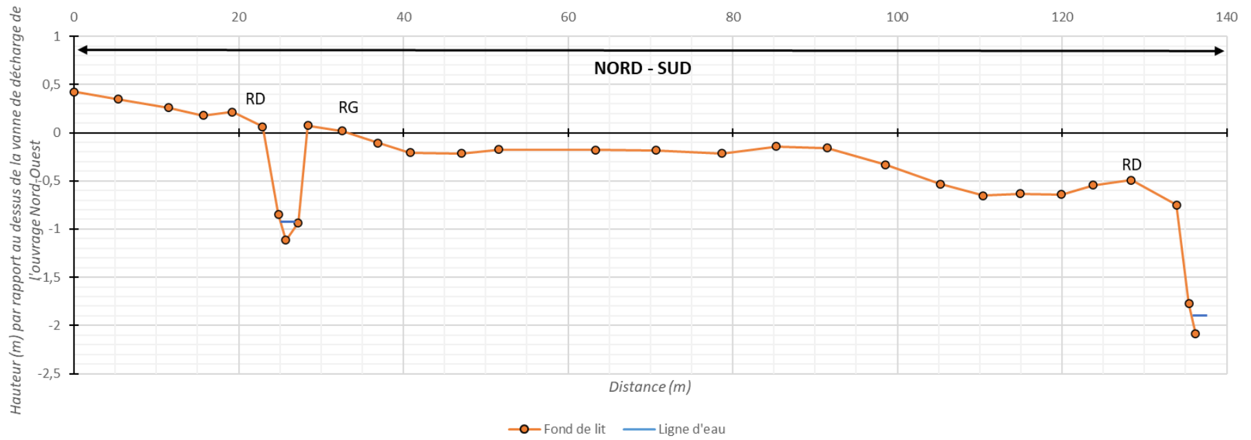
Profil en travers sur la Bondonne à Baugy Tronçon entre le bras Nord et le bras Sud de la Bondonne - 05/05
